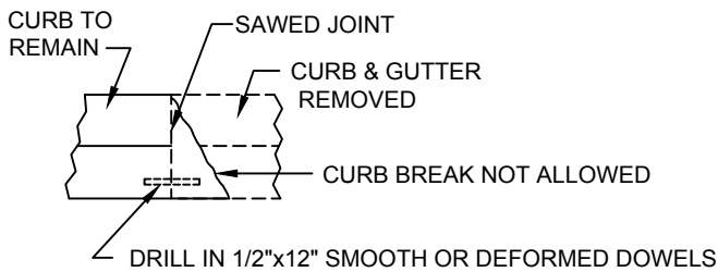
SECTION A2-A2
